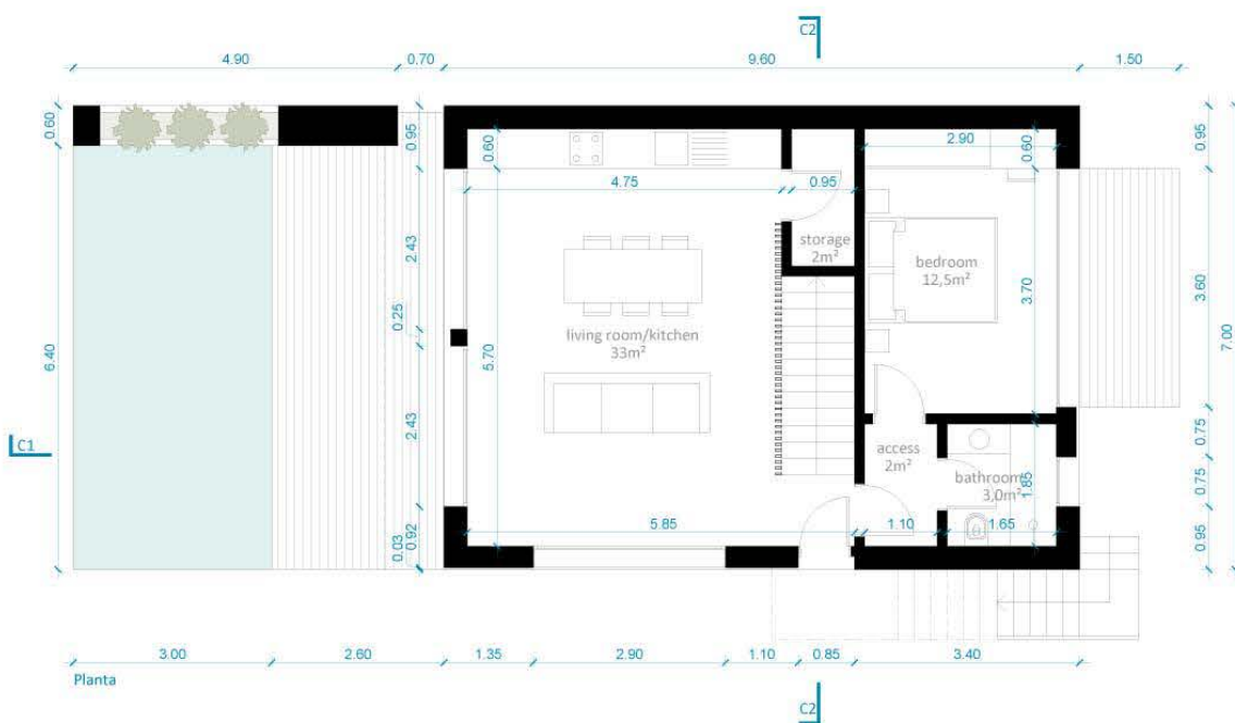
Planta Piso 1
